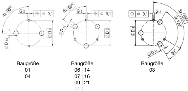
Bohrbild für Ankeraufnahme
